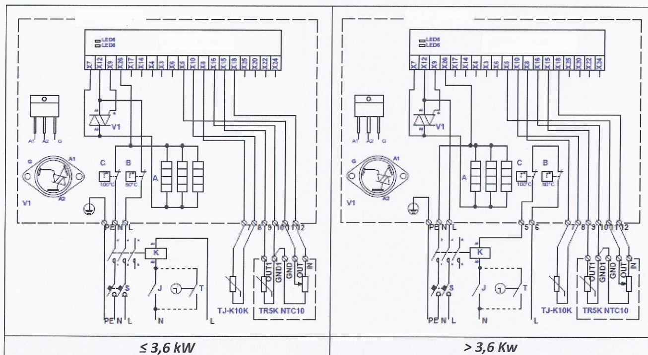
Fig. 62. Elektrische aansluitschema's van enkel fase 230V verwarmers KVE NI...-1f 2NTC
