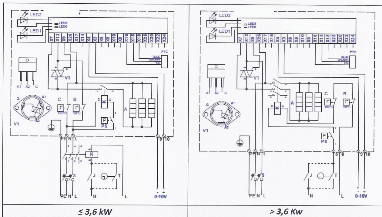
Fig. 83. Elektrische aansluitschema's van enkel fase 230V verwarmers KVE NIS...-...-1f PH
