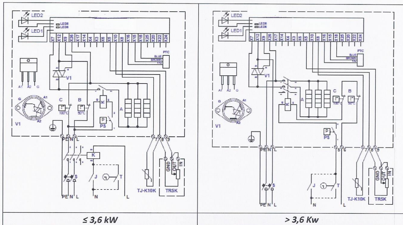
Fig. 59. Elektrische aansluitschema's van enkel fase 230V verwarmers KVE NI...-1f PH
