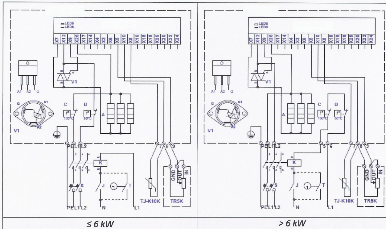
Fig. 45. Elektrische aansluitschema's van 2-fase 400V verwarmers KVE NI...-...-2f
