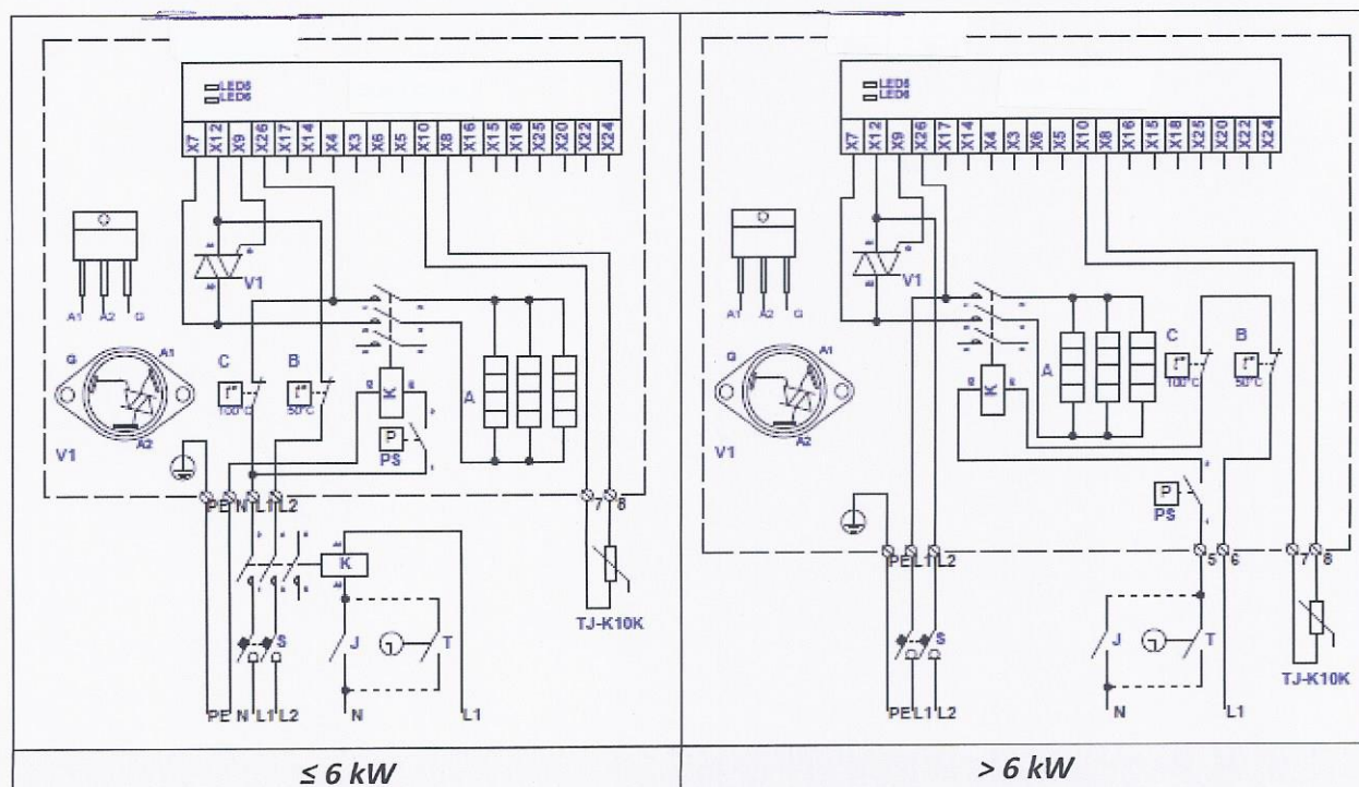
Fig. 24. Elektrische aansluitschema's van 2-fase 400V verwarmers KVE NV...-...-2f PS
