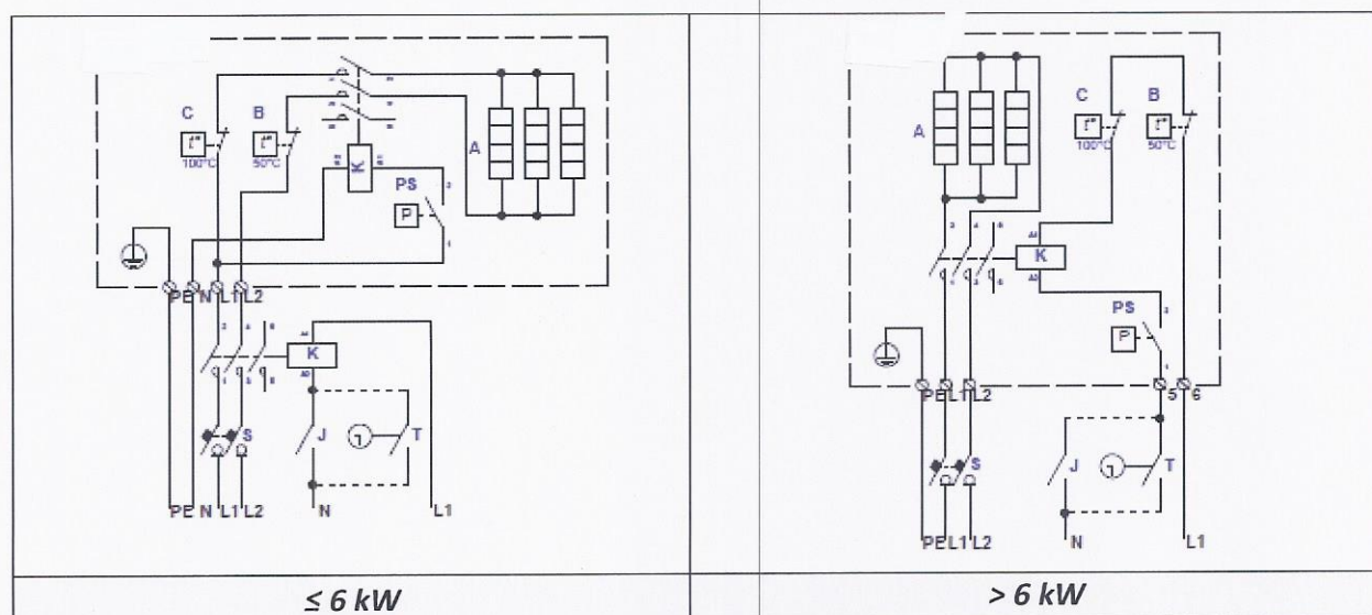
Fig. 18. Elektrische aansluitschema's van 2-fase 400V verwarmers KVE...-...-2f PS
