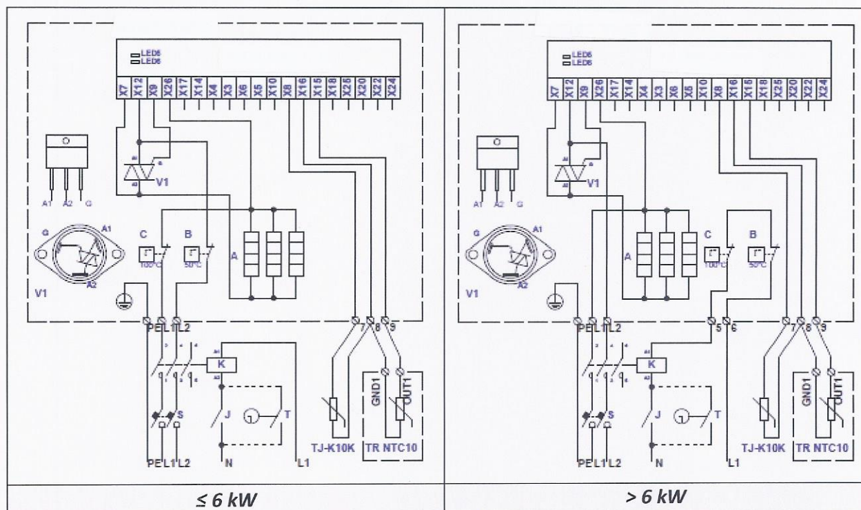
Fig. 39. Elektrische aansluitschema's van 2-fase 400V verwarmers KVE NV...-...-2f 2NTC
