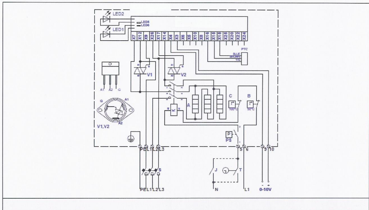
Fig. 79. Elektrisch aansluitschema van 3-fase 400V verwarmers KVE NIS....-3f PTC/PS
