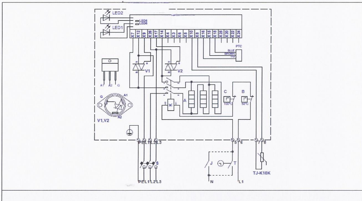
Fig. 34. Elektrisch aansluitschema van 3-fase 400V verwarmers KVE NV...-...-3f PTC/K
