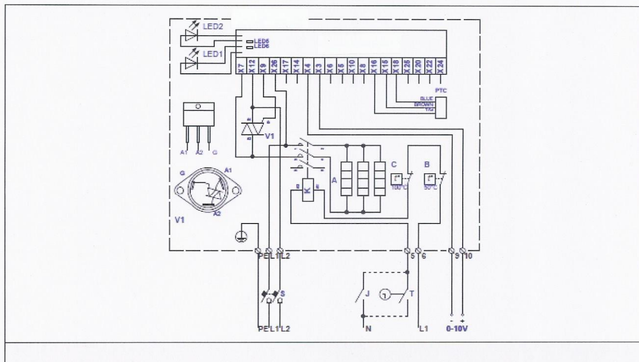
Fig. 81. Elektrisch aansluitschema van 2-fase 400V verwarmers KVE NIS...-...-2f PTC/K
