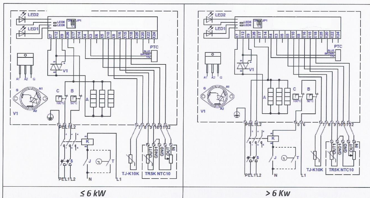
Fig. 66. Elektrische aansluitschema's van 2-fase 400V verwarmers KVE NI...-...-2f PTC/2NTC
