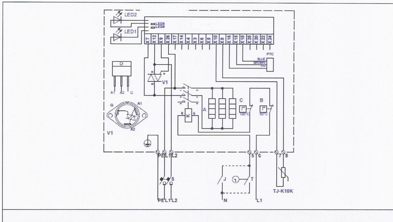
Fig. 33. Elektrisch aansluitschema van 2-fase 400V verwarmers KVE NV...-...-2f PTC/K
