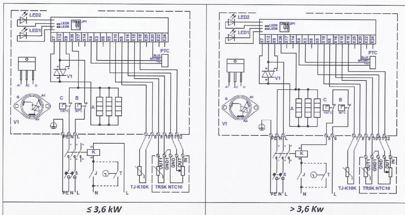
Fig. 65. Elektrische aansluitschema's van enkel fase 230V verwarmers KVE NI...-...-1f PTC/2NTC
