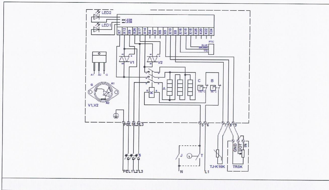
Fig. 58. Elektrisch aansluitschema van 3-fase 400V verwarmers KVE NI...-...-3f PTC/K
