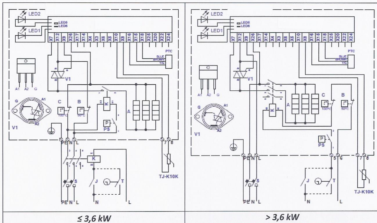
Fig. 29. Elektrische aansluitschema's van enkel fase 230V verwarmers KVE NV...-1f PTC/PS
