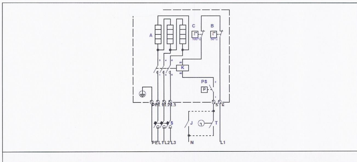
Fig. 19. Elektrisch aansluitschema van 3-fase 400V verwarmers KVE...-...-3f PS
