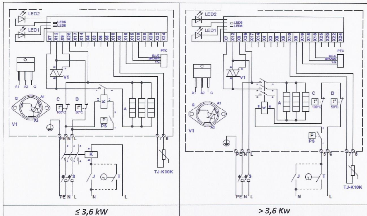
Fig. 35. Elektrische aansluitschema's van enkel fase 230V verwarmers KVE NV...-...-1f PH
