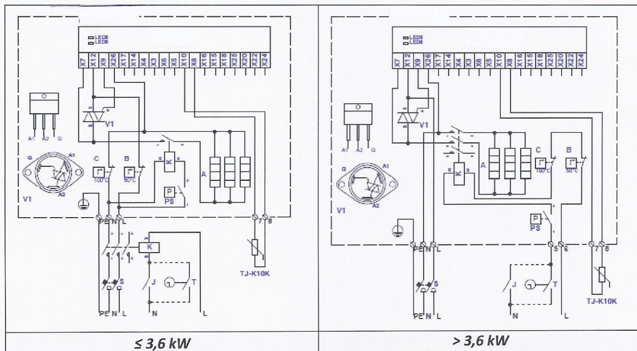
Fig. 23. Elektrische aansluitschema's van enkel fase 230V verwarmers KVE NV...-...-1f PS
