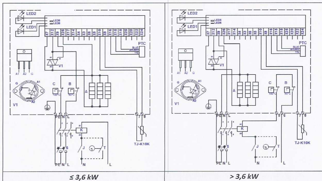
Fig. 26. Elektrische aansluitschema's van enkel fase 230V verwarmers KVE NV...-1f PTC
