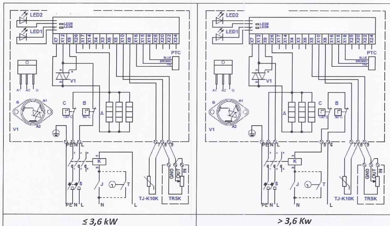
Fig. 50. Elektrische aansluitschema's van enkel fase 230V verwarmers KVE NI...-...-1f PTC
