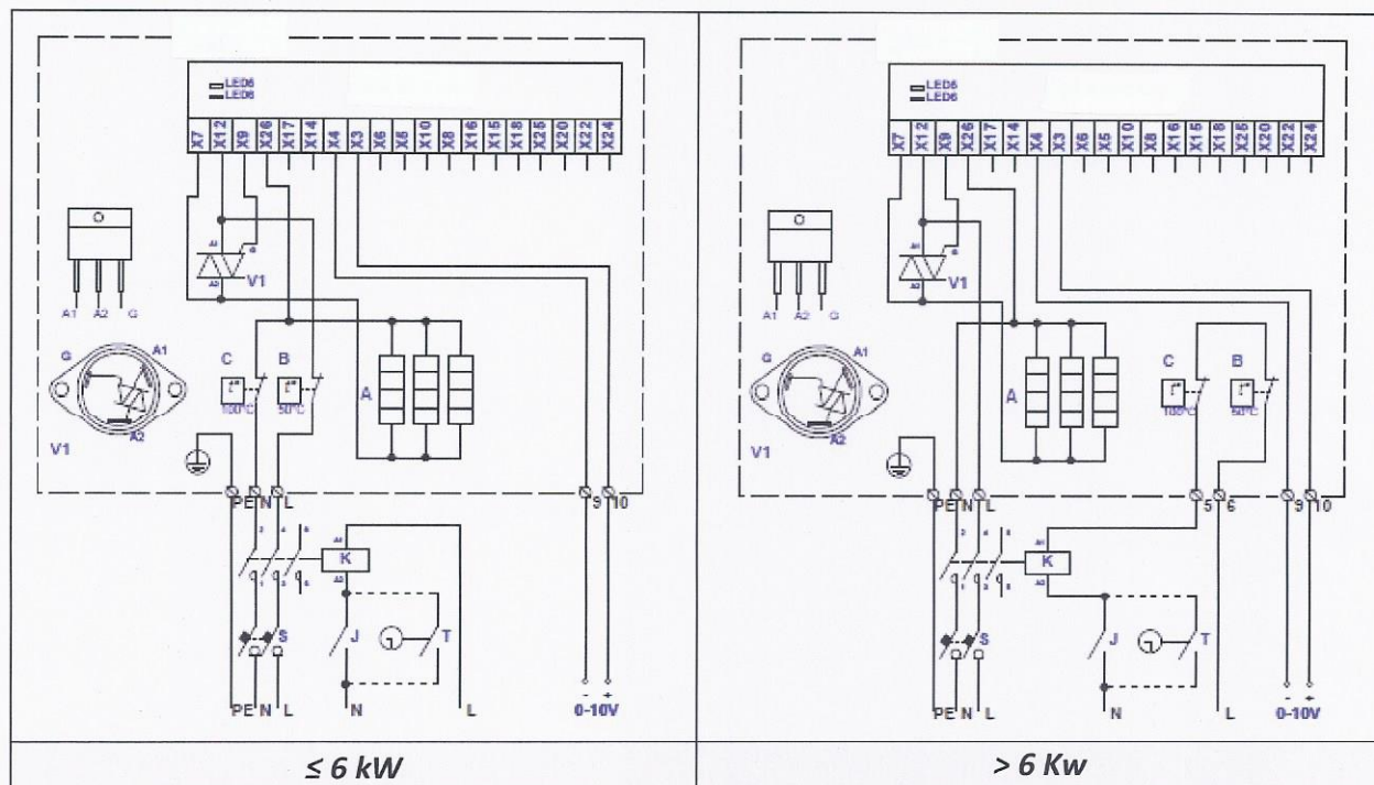
Fig. 69. Elektrische aansluitschema's van 2-fase 400V verwarmers KVE NIS...-...-2f
