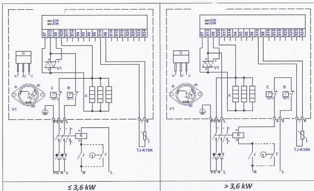
Fig. 20. Elektrische aansluitschema's van enkel fase 230V verwarmers KVE NV...-...-1f
