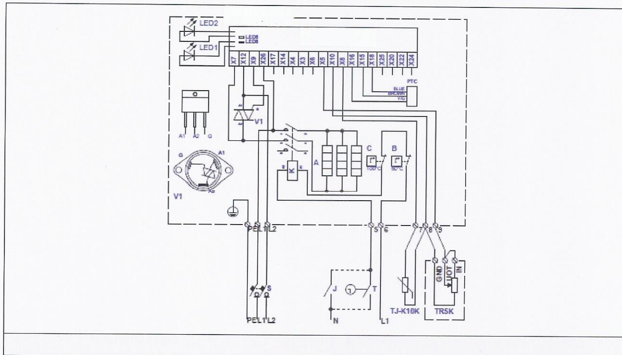
Fig. 57. Elektrisch aansluitschema van 2-fase 400V verwarmers KVE NI...-...-2f PTC/K
