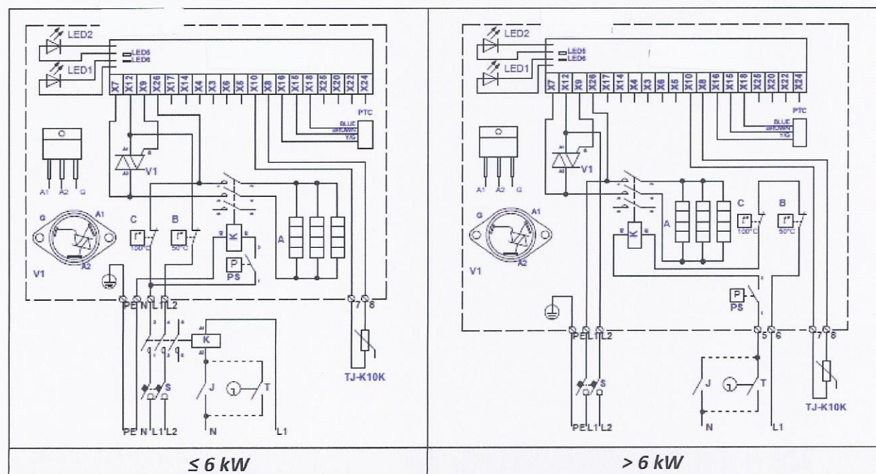
Fig. 36. Elektrische aansluitschema's van 2-fase 400V verwarmers KVE NV...-...-2f PH
