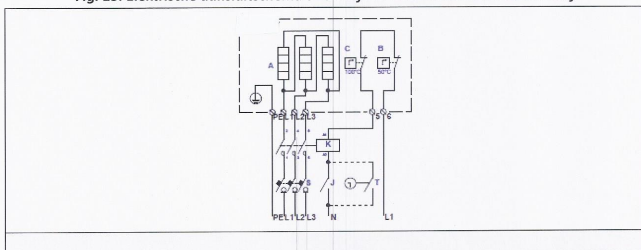
Fig. 16. Elektrisch aansluitschema van 3-fase 400V verwarmers KVE.....-3f
