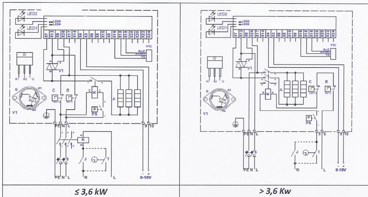
Fig. 77. Elektrische aansluitschema's van enkel fase 230V verwarmers KVE NIS...-...-1f PTC/PS
