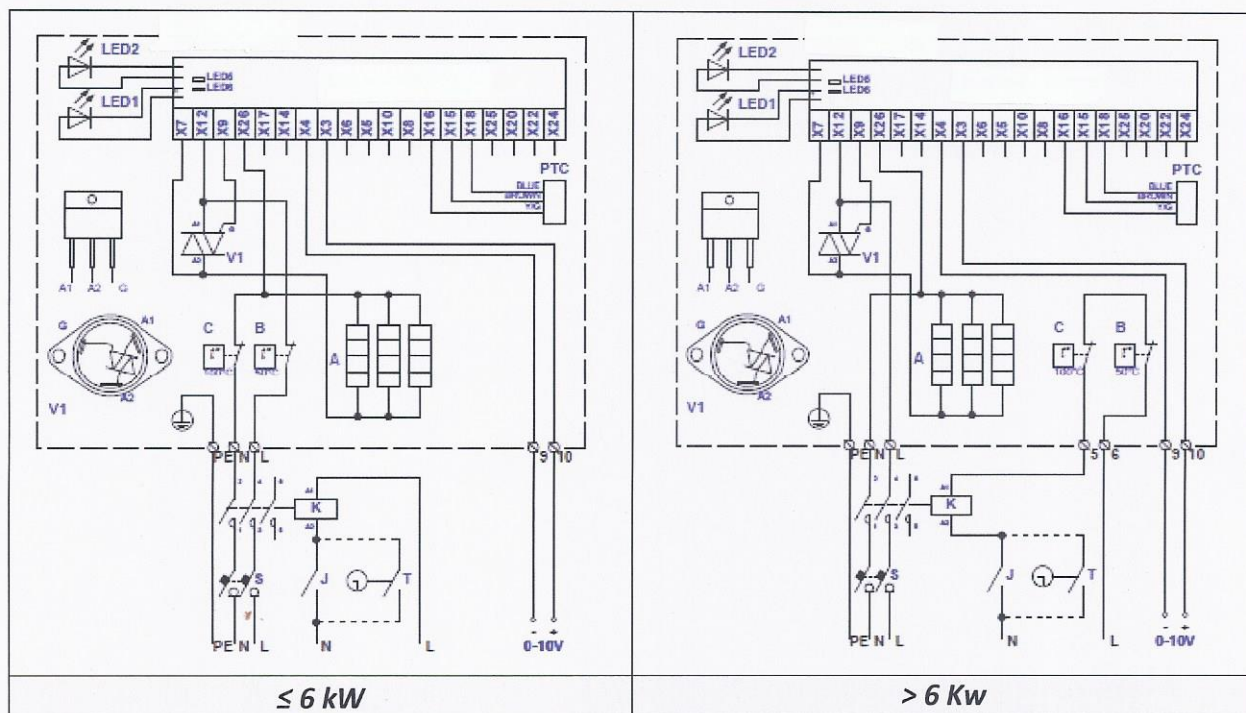
Fig. 75. Elektrische aansluitschema's van 2-fase 400V verwarmers KVE NIS...-...-2f PTC
