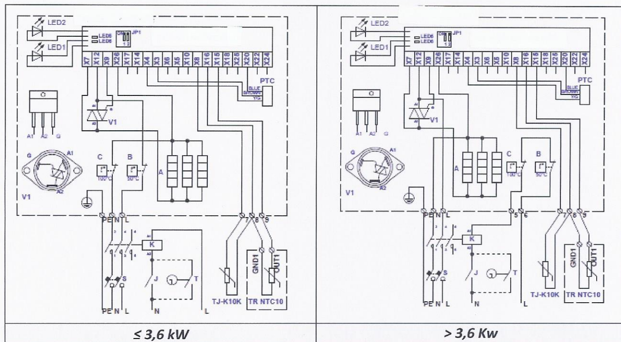
Fig. 41. Elektrische aansluitschema's van enkel fase 230V verwarmers KVE NV...-...-1f PTC/2NTC
