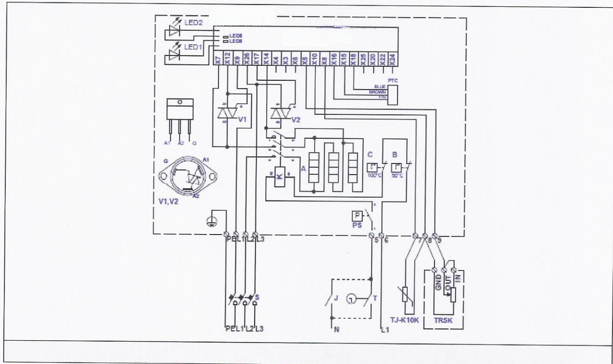
Fig. 55. Elektrisch aansluitschema van 3-fase 400V verwarmers KVE NI...-...-3f PTC/PS
