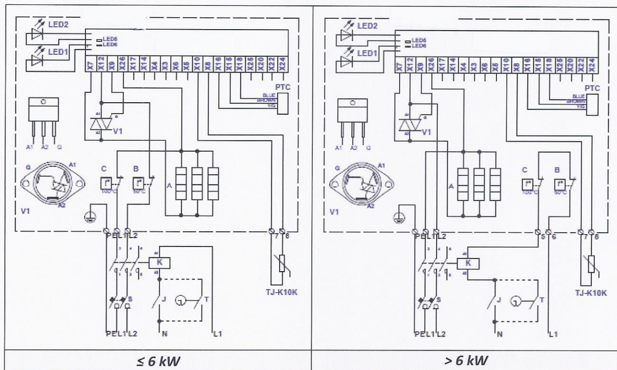
Fig. 27. Elektrische aansluitschema's van 2-fase 400V verwarmers KVE NV...-...-2f PTC
