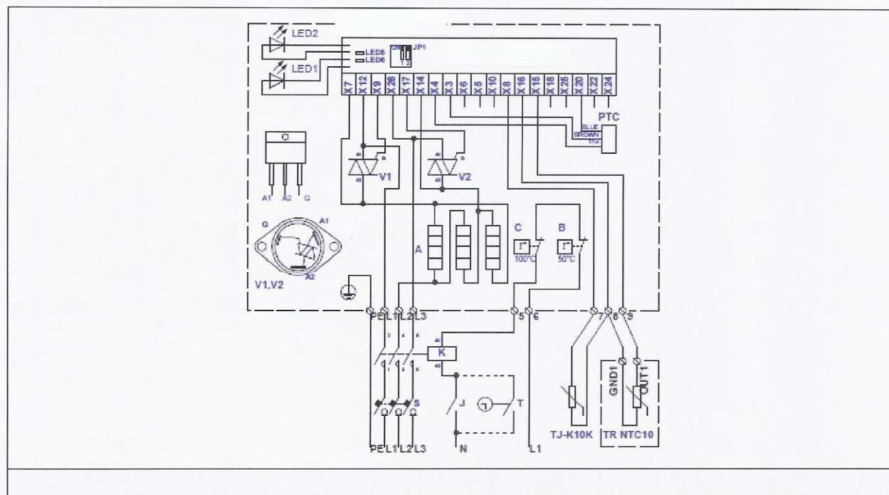
Fig. 43. Elektrisch aansluitschema van 3-fase 400V verwarmers KVE NV...-...-3f PTC/2NTC
