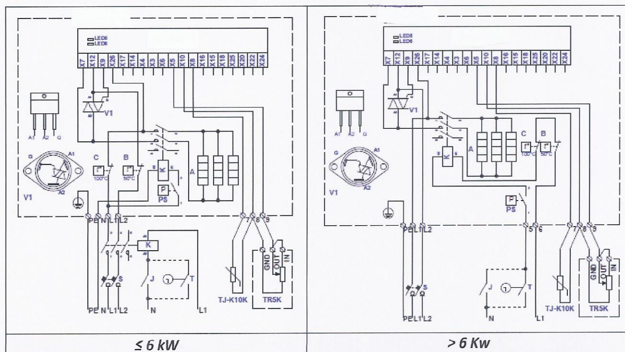
Fig. 48. Elektrische aansluitschema's van 2-fase 400V verwarmers KVE NI...-...-2f PS
