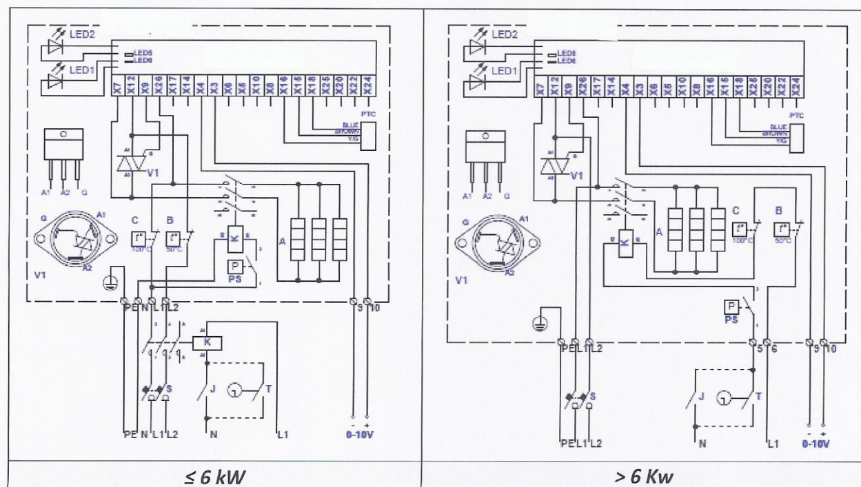
Fig. 84. Elektrische aansluitschema's van 2-fase 400V verwarmers KVE NIS...-...-2f PH
