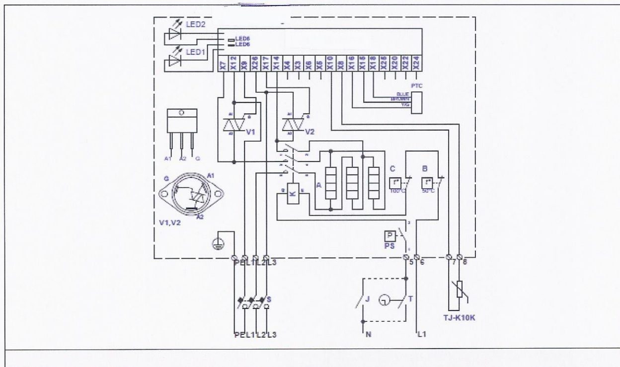
Fig. 31. Elektrisch aansluitschema van 3-fase 400V verwarmers KVE NV...-...-3f PTC/PS
