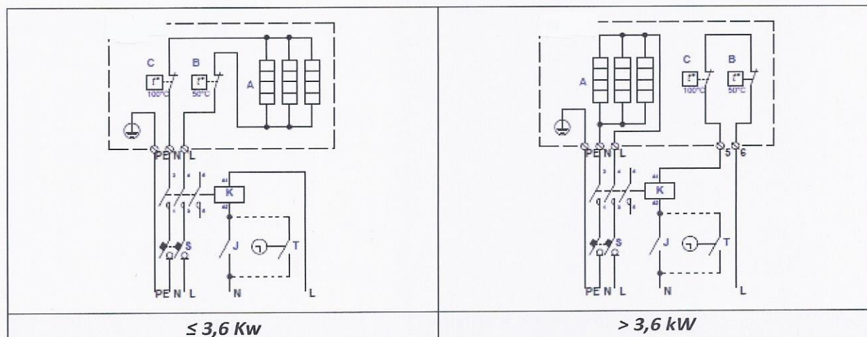
Fig. 14. Elektrisch aansluitschema van enkel fase 230V verwarmers KVE...-1f
