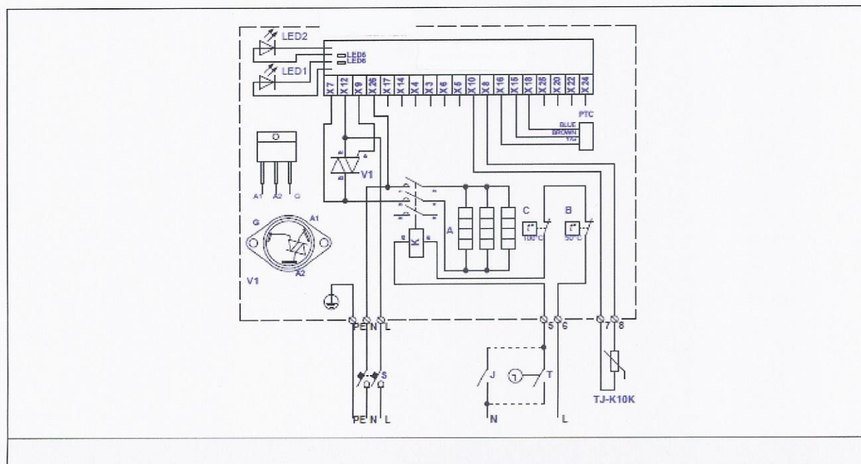
Fig. 32. Elektrisch aansluitschema van enkel fase 230V verwarmers KVE NV...-...-1f PTC/K
