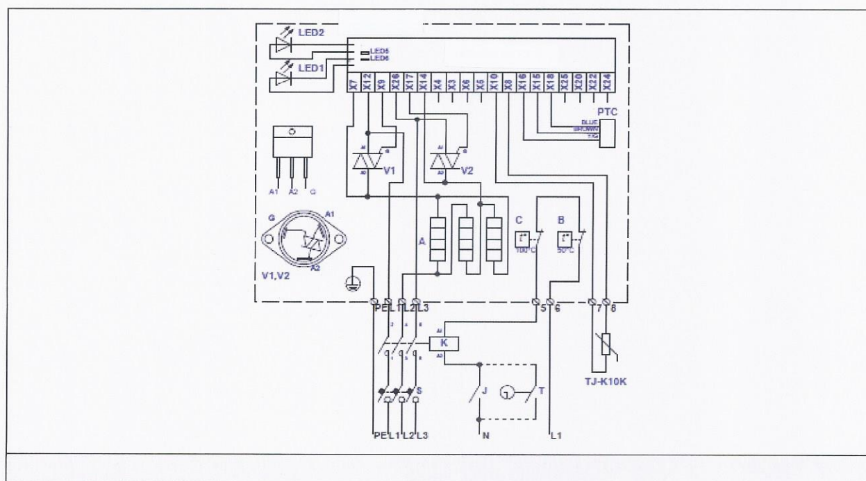
Fig. 28. Elektrisch aansluitschema van 3-fase 400V verwarmers KVE NV...-...-3f PTC
