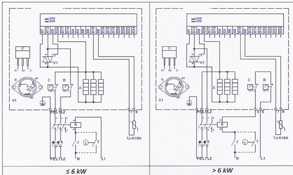
Fig. 21. Elektrische aansluitschema's van 2-fase 400V verwarmers KVE NV...-...-2f
