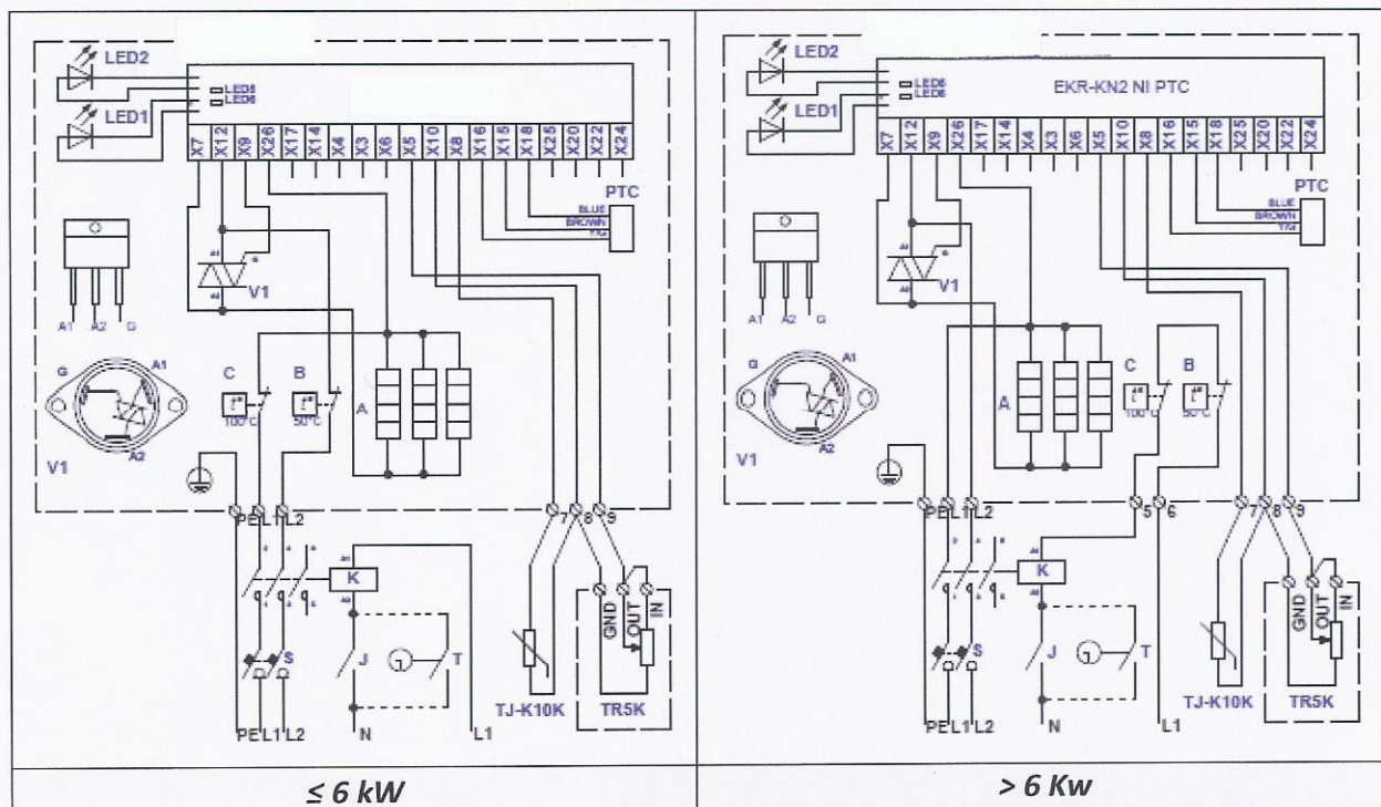
Fig. 51. Elektrische aansluitschema's van 2-fase 400V verwarmers KVE NI...-2f PTC
