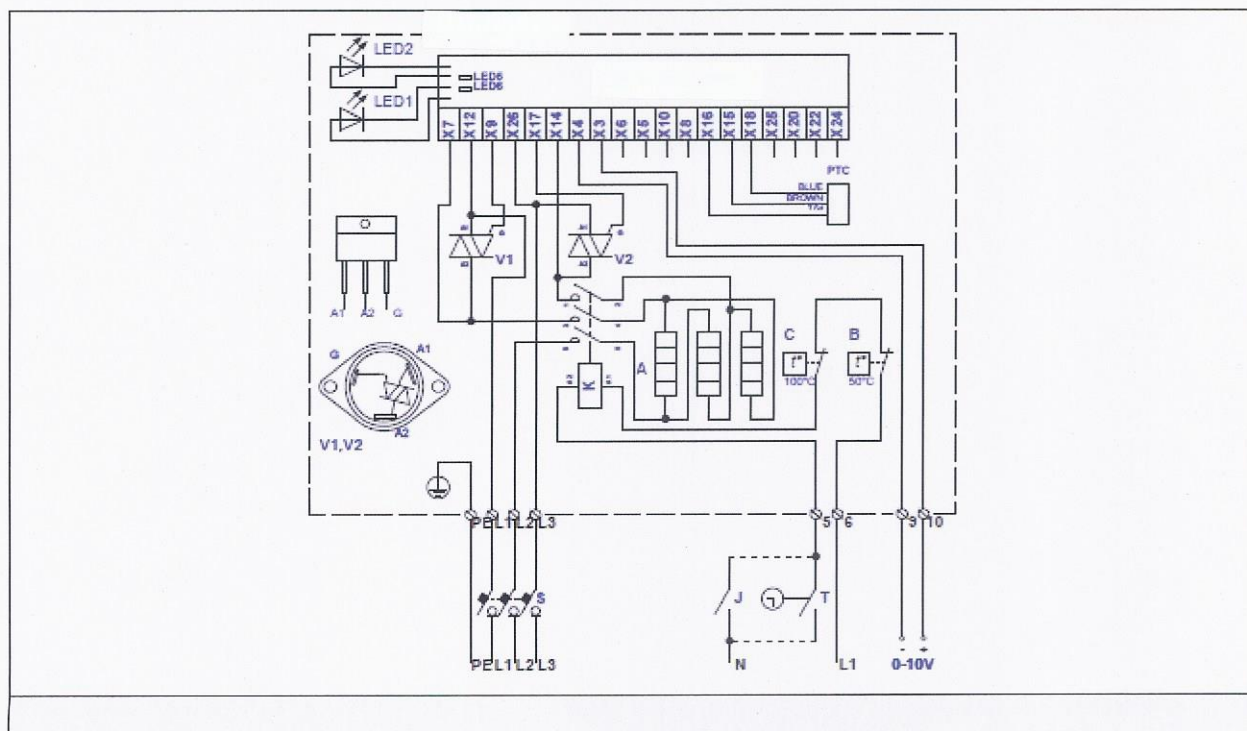
Fig. 82. Elektrisch aansluitschema van 3-fase 400V verwarmers KVE NIS...-...-3f PTC/K
