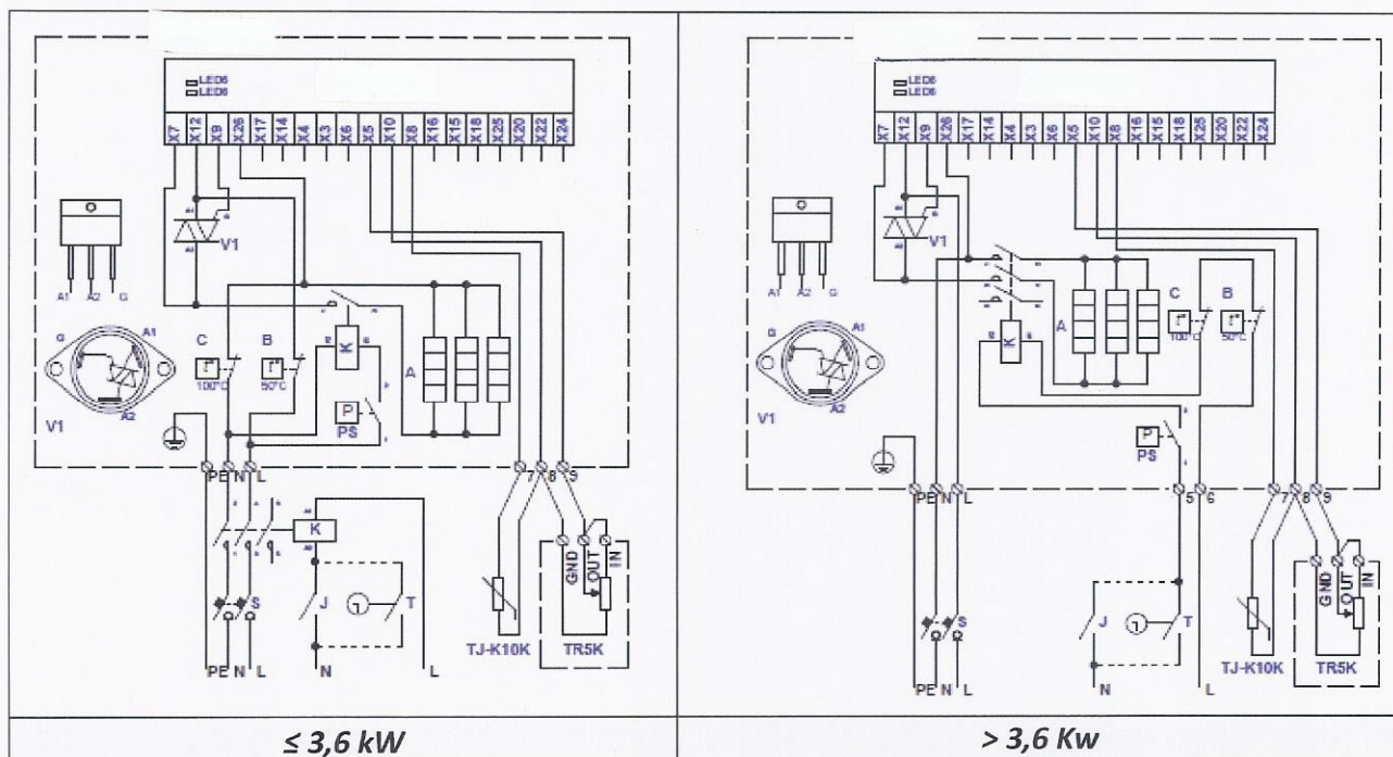
Fig. 47. Elektrische aansluitschema's van enkel fase 230V verwarmers KVE NI...-...-1f PS
