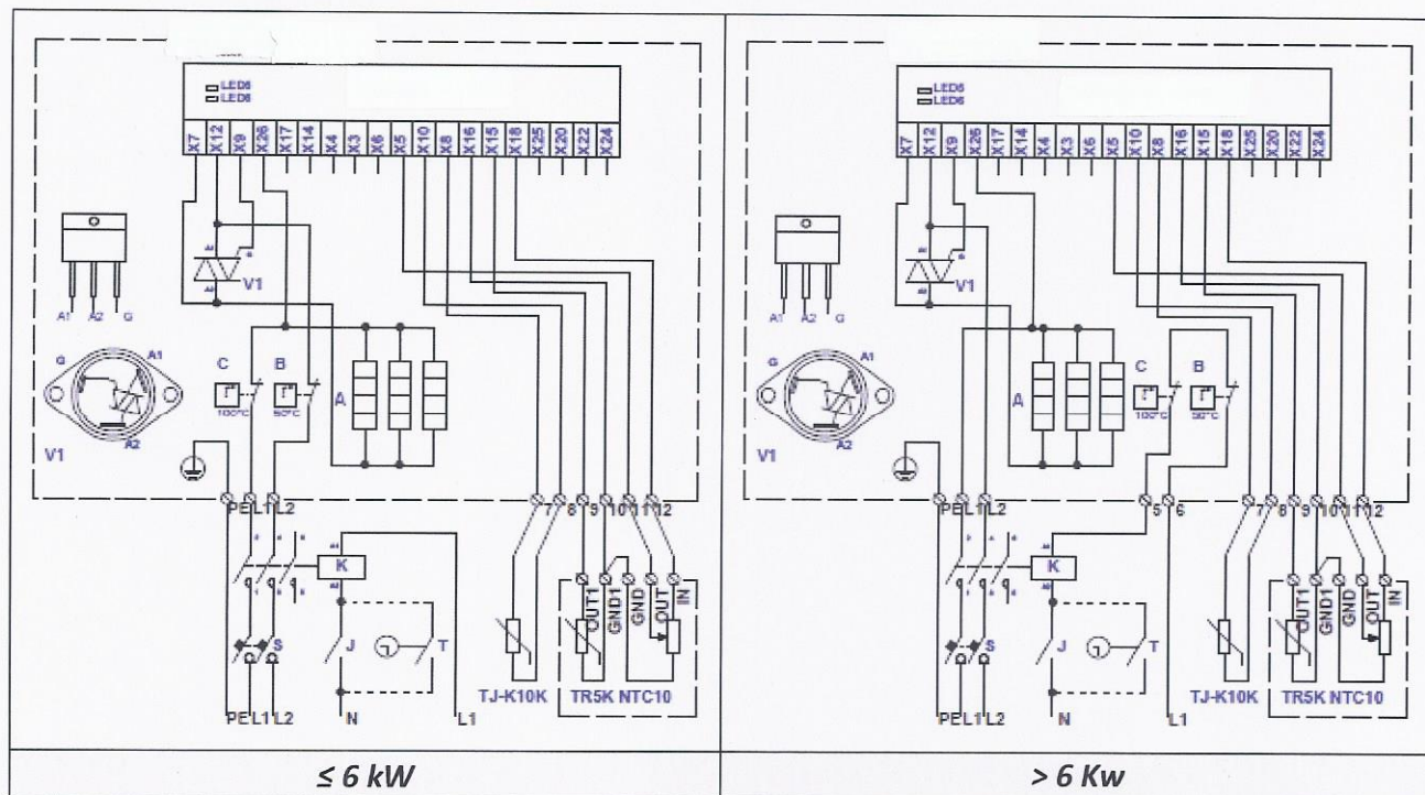
Fig. 63. Elektrische aansluitschema's van 2-fase 400V verwarmers KVE NI...-...-2f 2NTC
