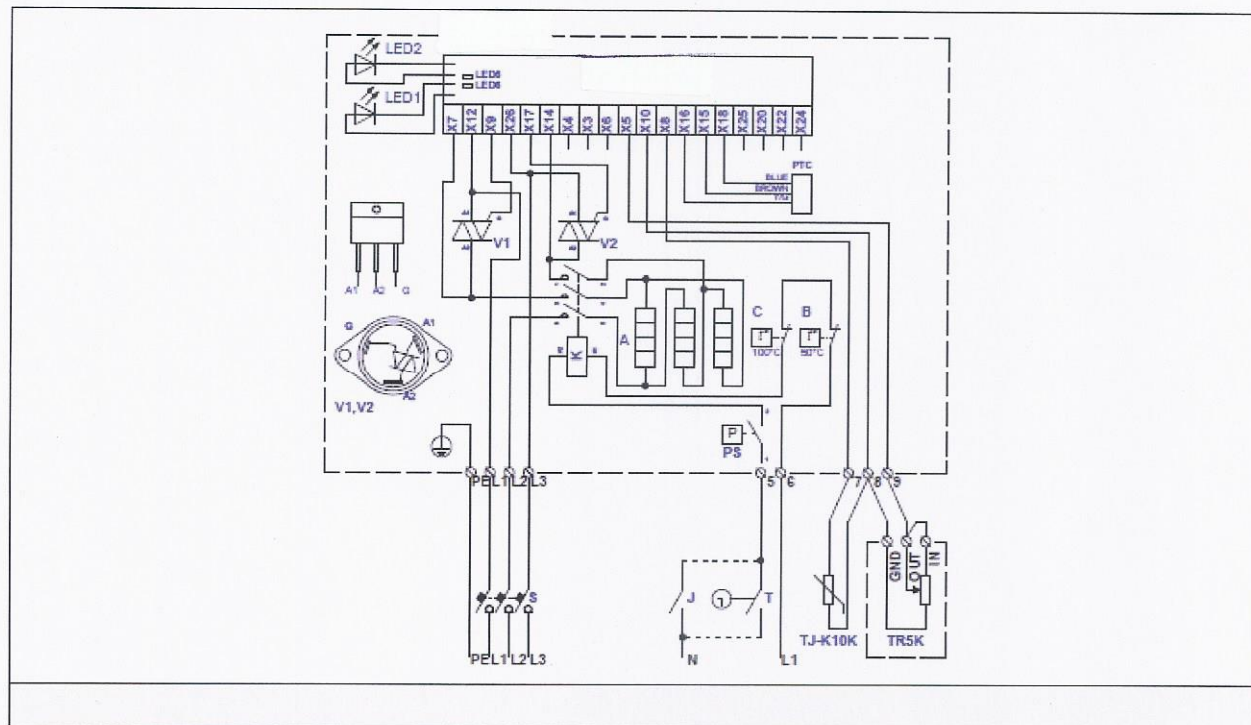
Fig. 61. Elektrisch aansluitschema van 3-fase 400V verwarmers KVE NI...-3f PH
