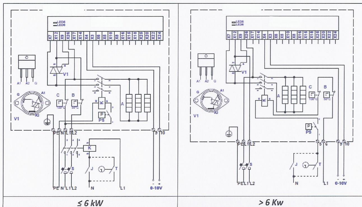
Fig. 72. Elektrische aansluitschema's van 2-fase 400V verwarmers KVE NIS...-...-2f PS
