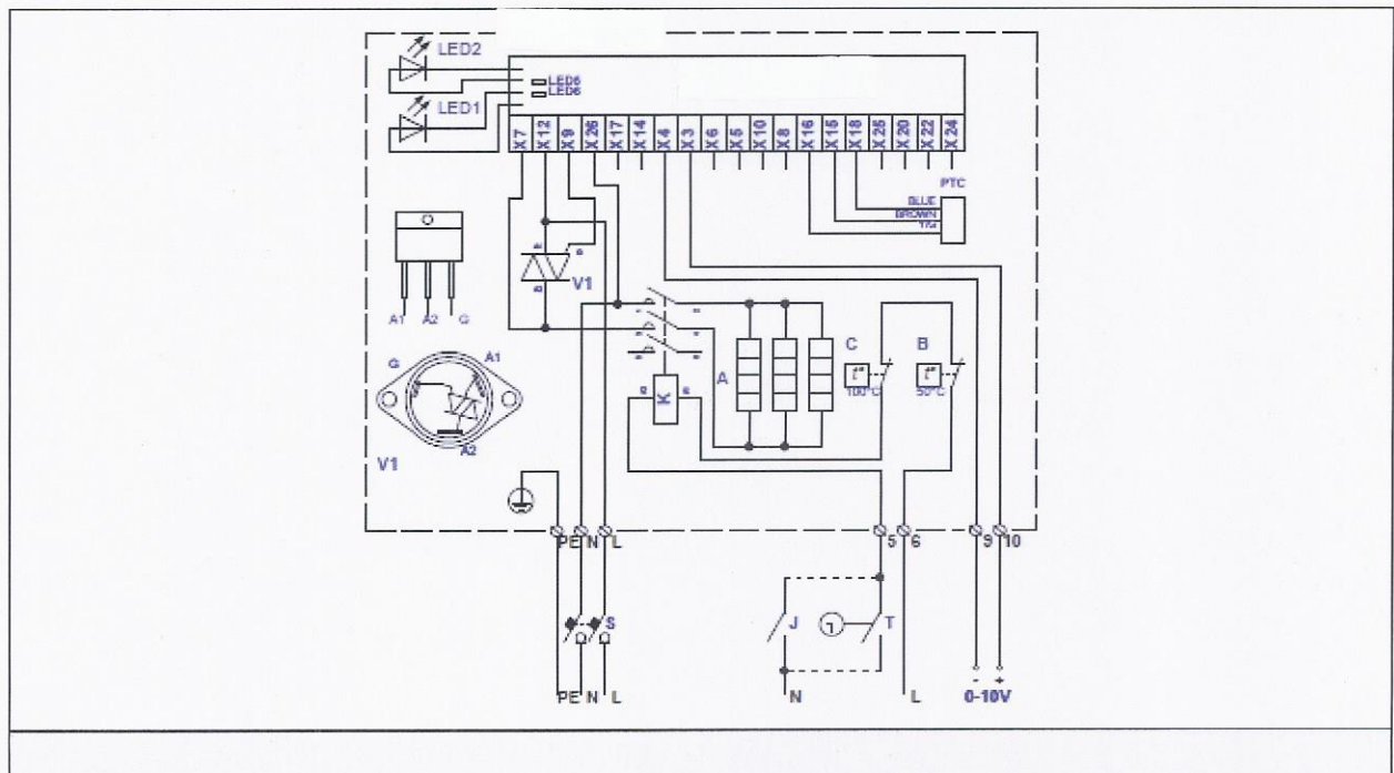
Fig. 80. Elektrisch aansluitschema van enkel fase 230V verwarmers KVE NIS....-1f PTC/K
