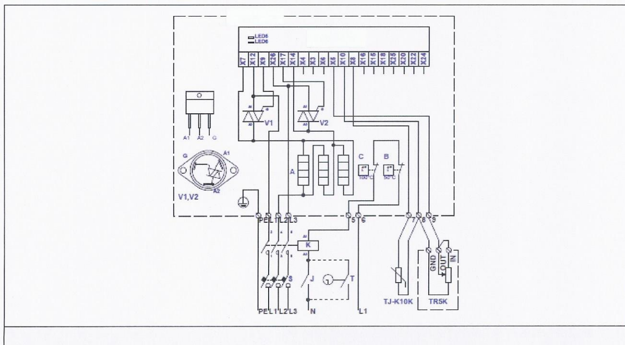
Fig. 46. Elektrisch aansluitschema van 3-fase 400V verwarmers KVE NI...-...-3f
