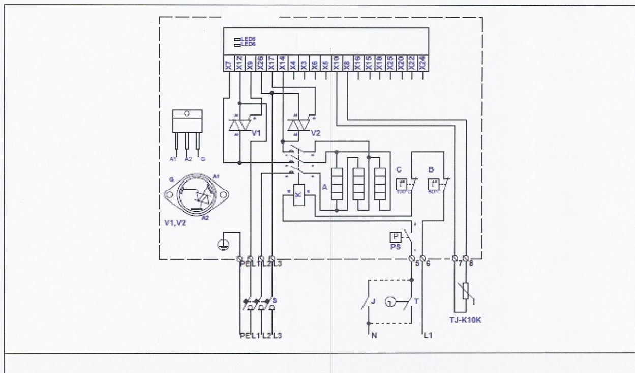
Fig. 25. Elektrisch aansluitschema van 3-fase 400V verwarmers KVE NV...-3f PS
