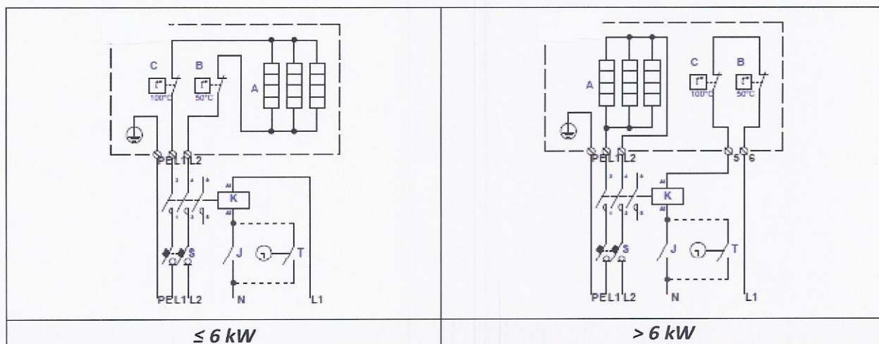
Fig. 15. Elektrische aansluitschema's van 2-fase 400V verwarmers KVE.....-2f
