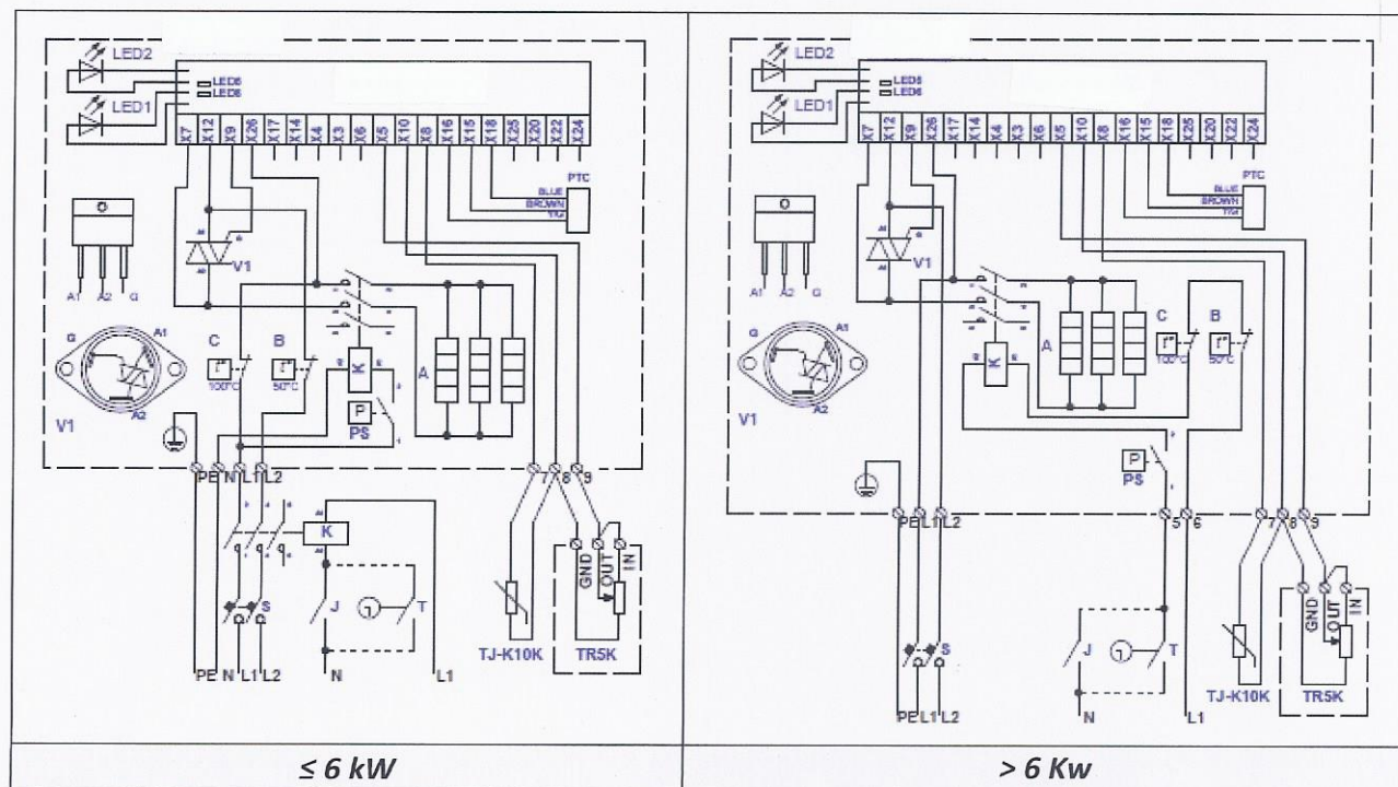
Fig. 60. Elektrische aansluitschema's van 2-fase 400V verwarmers KVE NI...-2f PH
