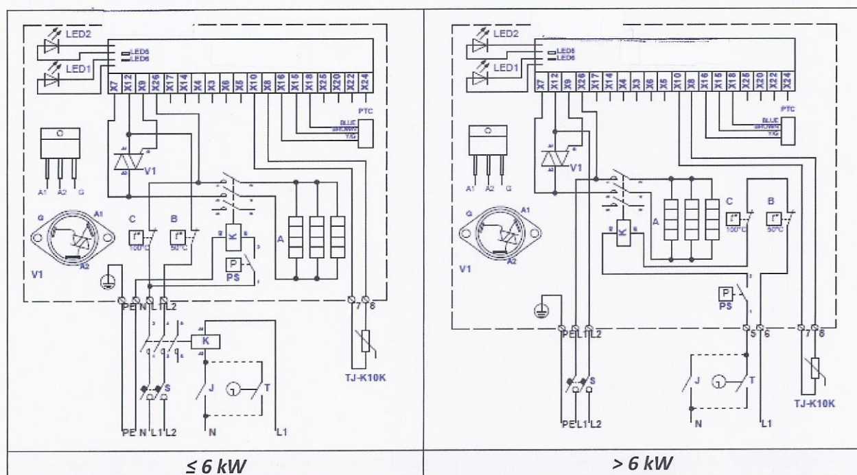
Fig. 30. Elektrische aansluitschema's van 2-fase 400V verwarmers KVE NV...-2f PTC/PS
