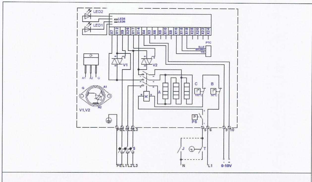
Fig. 85. Elektrisch aansluitschema van 3-fase 400V verwarmers KVE NIS...-...-3f PH
