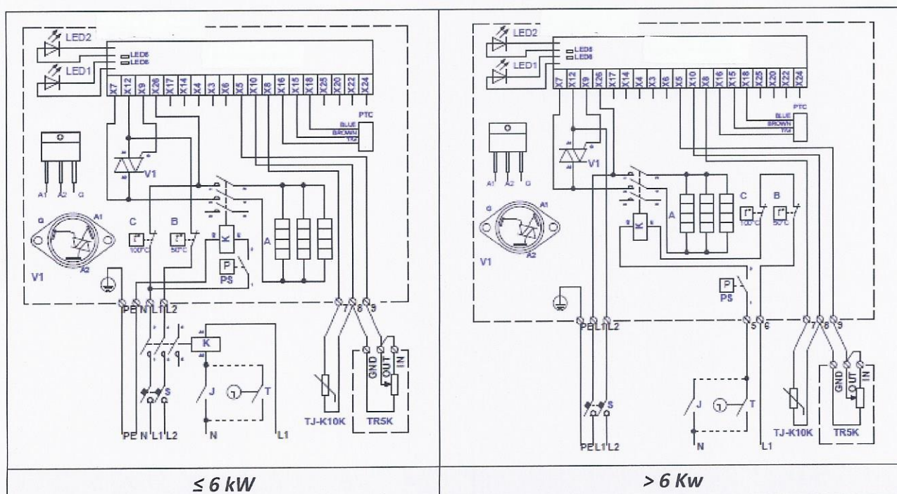
Fig. 54. Elektrische aansluitschema's van 2-fase 400V verwarmers KVE NI...-...-2f PTC/PS
