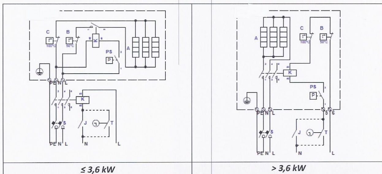
Fig. 17. Elektrische aansluitschema's van enkel fase 230V verwarmers KVE...-...-1f PS
