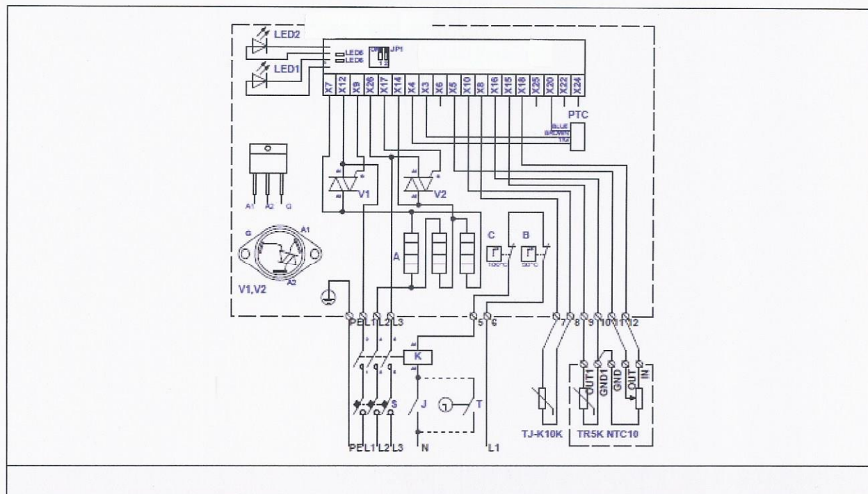
Fig. 67. Elektrisch aansluitschema van 3-fase 400V verwarmer KVE NI...-...-3f PTC/2NTC
