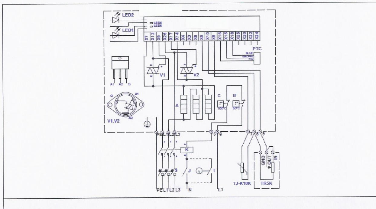
Fig. 52. Elektrisch aansluitschema van 3-fase 400V verwarmers KVE NI...-3f PTC
