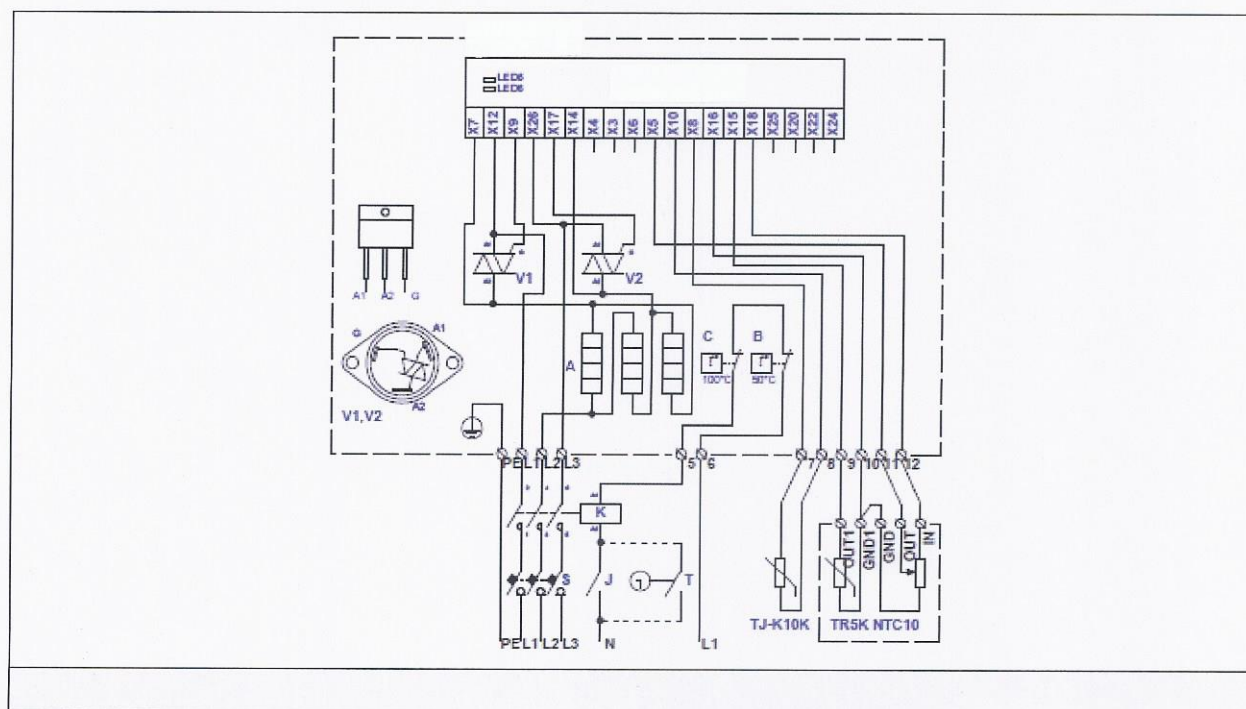
Fig. 64. Elektrisch aansluitschema van 3-fase 400V verwarmers KVE NI...-...-3f 2NTC
