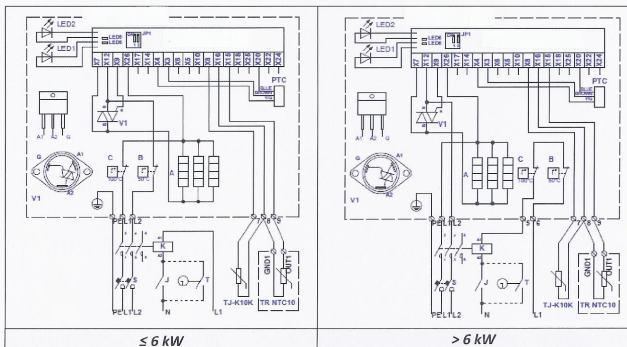
Fig. 42. Elektrische aansluitschema's van 2-fase 400V verwarmers KVE NV...-...-2f PTC/2NTC
