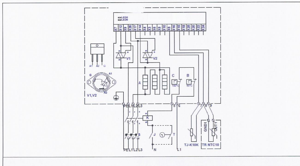
Fig. 40. Elektrisch aansluitschema van 3-fase 400V verwarmers KVE NV...-...-3f 2NTC
