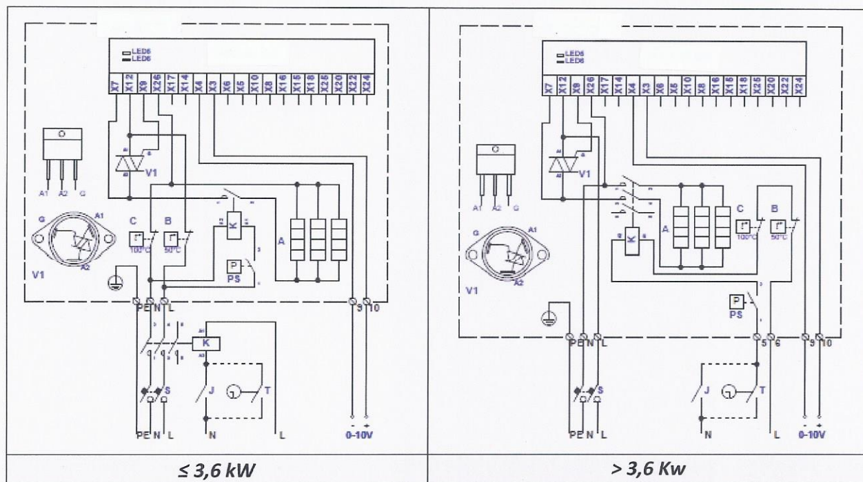
Fig. 71. Elektrische aansluitschema's van enkel fase 230V verwarmers KVE NIS...-...-1f PS
