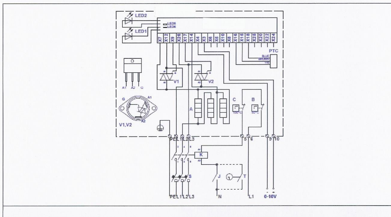
Fig. 76. Elektrisch aansluitschema van 3-fase 400V verwarmers KVE NIS...-...-3f PTC
