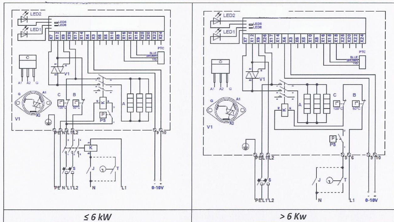
Fig. 78. Elektrische aansluitschema's van 2-fase 400V verwarmers KVE NIS...-...-2f PTC/PS
