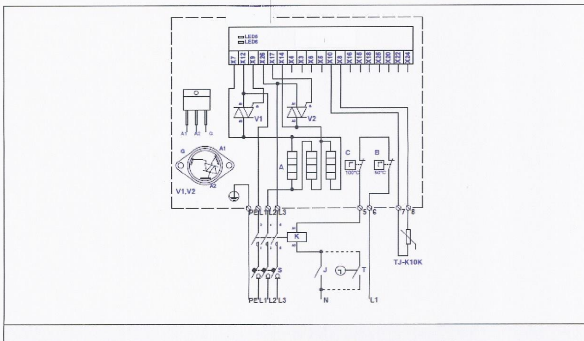
Fig. 22. Elektrisch aansluitschema van 3-fase 400V verwarmers KVE NV...-...-3f
