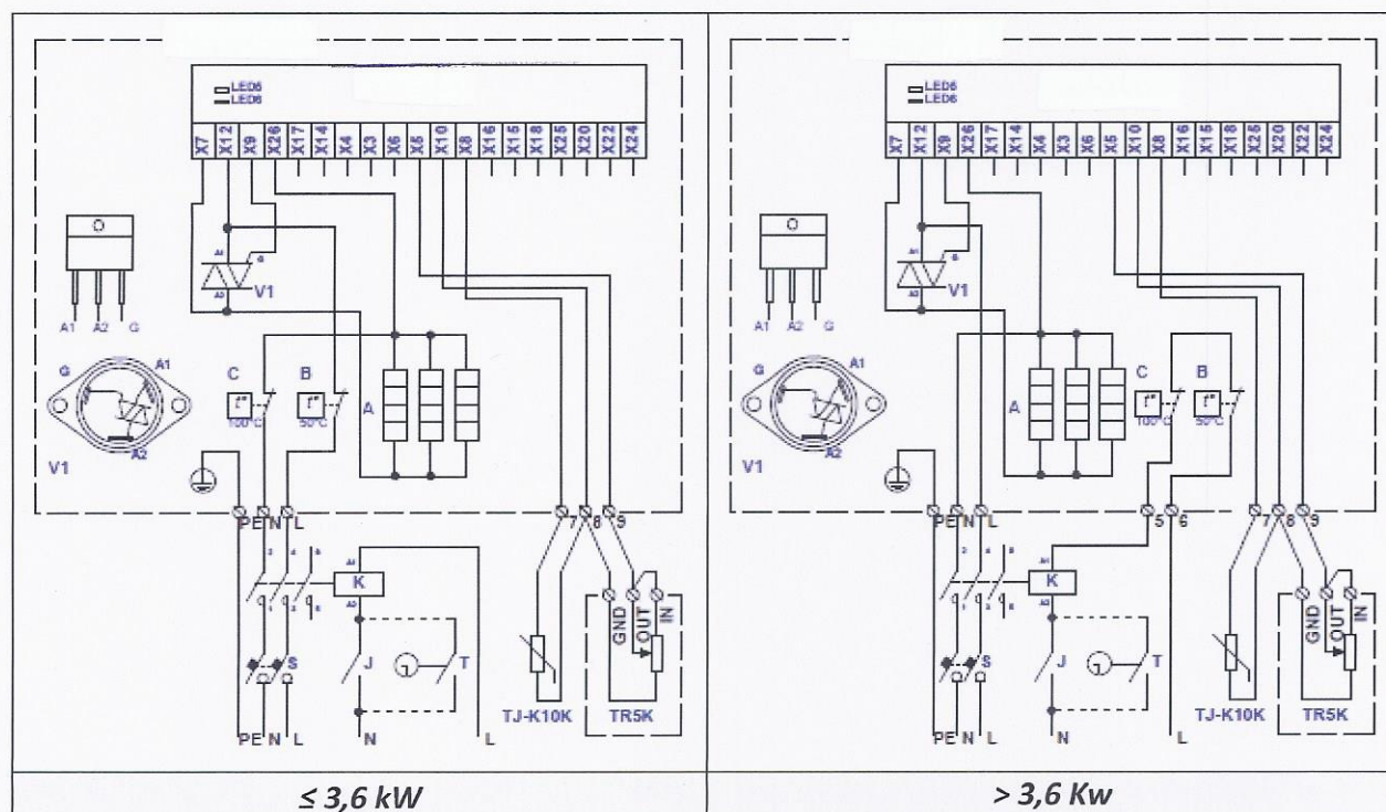
Fig. 44. Elektrische aansluitschema's van enkel fase 230V verwarmers KVE NI...-...-1f
