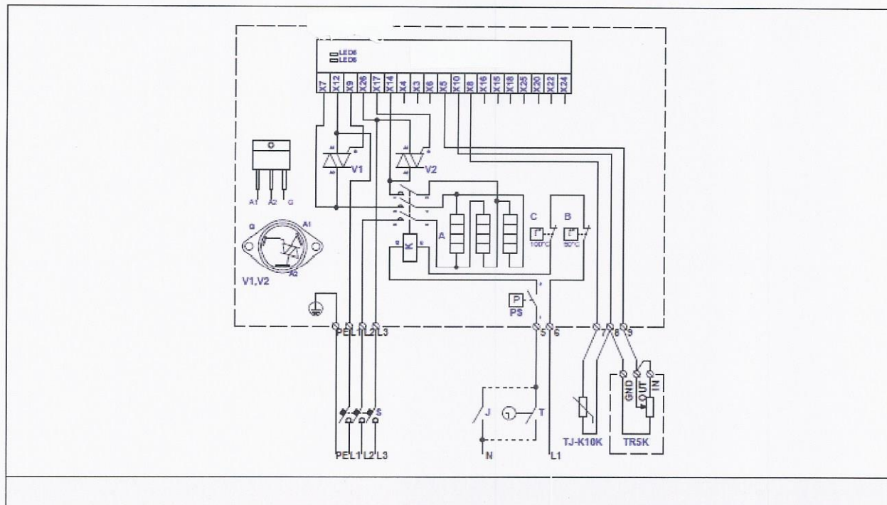
Fig. 49. Elektrisch aansluitschema van 3-fase 400V verwarmers KVE NI...-...-3f PS
