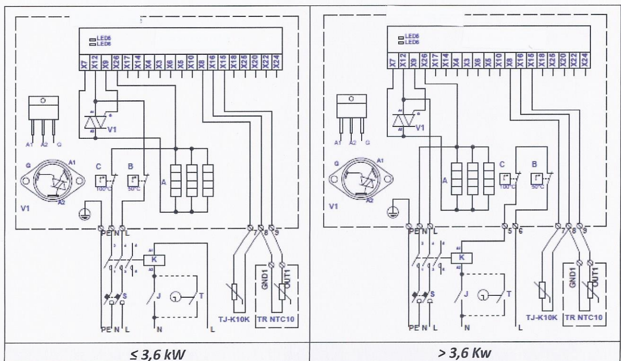
Fig. 38. Elektrische aansluitschema's van enkel fase 230V verwarmer KVE NV...-...-1f 2NTC
