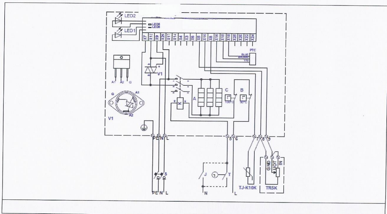
Fig. 56. Elektrisch aansluitschema van enkel fase 230V verwarmers KVE NI...-...-1f PTC/K
