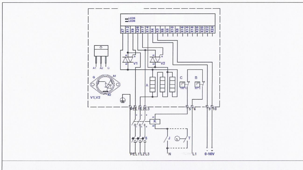
Fig. 70. Elektrisch aansluitschema van 3-fase 400V verwarmers KVE NIS...-...-3f
