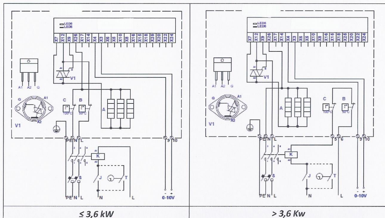
Fig. 68. Elektrische aansluitschema's van enkel fase 230V verwarmers KVE NIS...-...-1f
