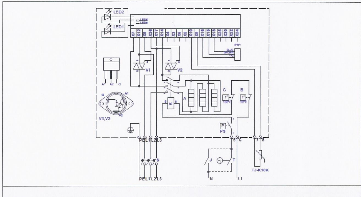
Fig. 37. Elektrisch aansluitschema van 3-fase 400V verwarmer KVE NV...-...-3f PH
