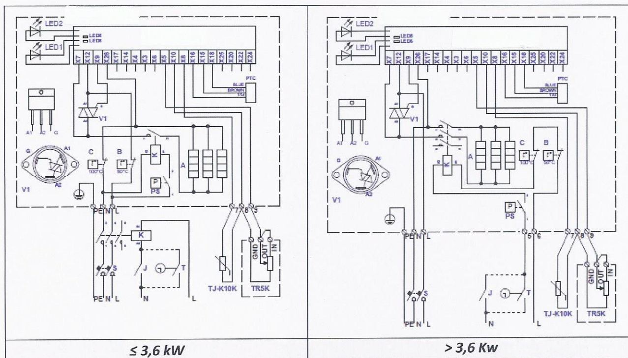
Fig. 53. Elektrische aansluitschema's van enkel fase 230V verwarmers KVE NI...-...-1f PTC/PS
