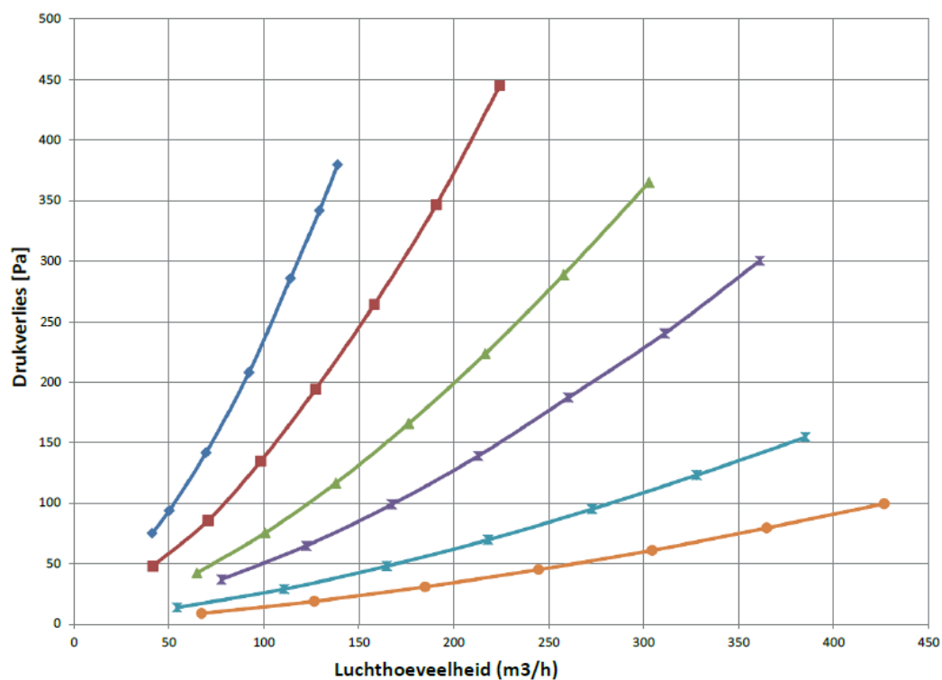
Grafiek met drukverlies
